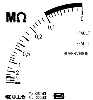
Abb. 2, 10...0MΩ Skala
