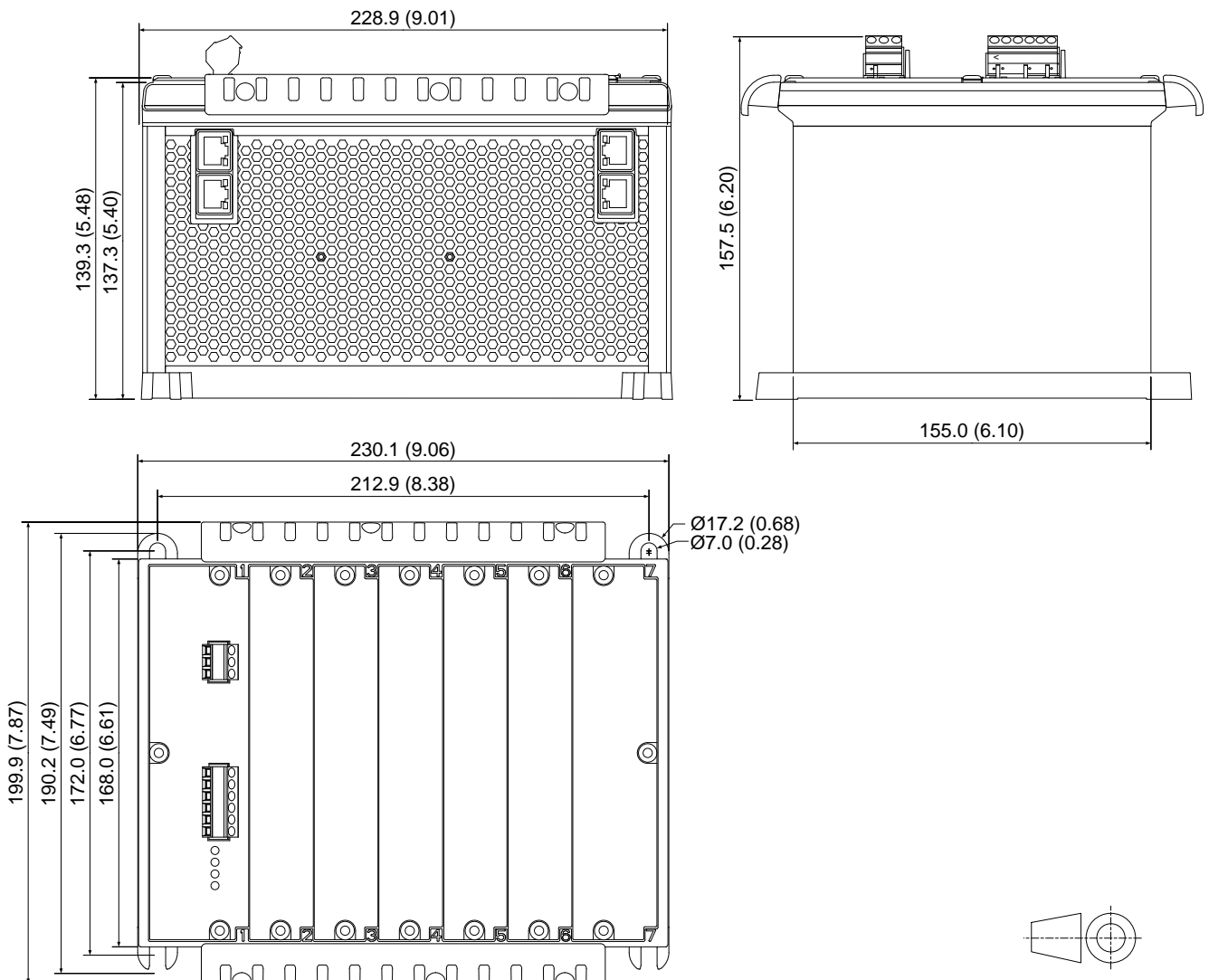
Figure 3.1 Le rack R7.1 avec dimensions en mm (et dimensions approximatives en pouces), projection premier angle, comprend le module PSM3.1 et des caches
