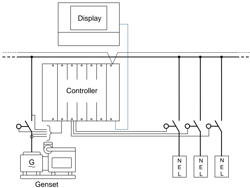
Figure 1.1 Exemple d'une application de contrôleur, avec les charges non-essentiels en option
