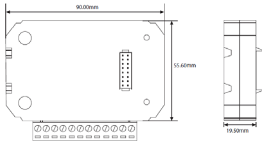
Габаритные размеры модуля входов/выходов
