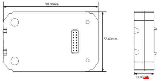
Габаритные размеры коммуникационного модуля
