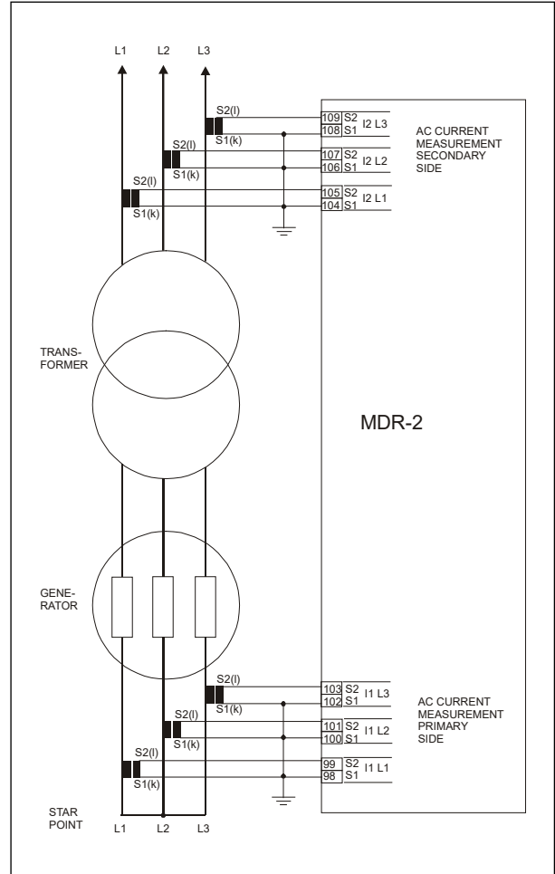
Diagramme de principe, option C4
