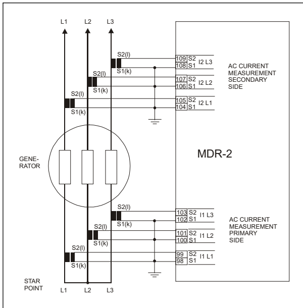
Diagramme de principe
